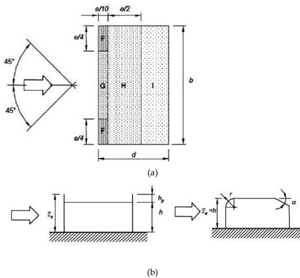
a) Suddivisione delle coperture piane in zone di uguale pressione,
